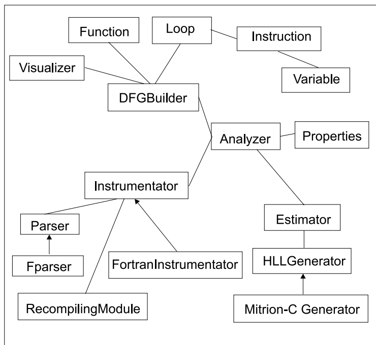
Rys. 3. Diagram klas
