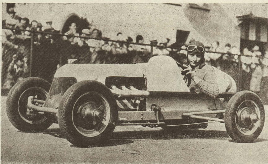
Młody technik amerykański Don Arlen zaprojektował i własnoręcznie wykonał miniaturowy samochód, posiadający powietrzne chłodzenie silnika i napęd na przednie koła. Podobno wózek ten ma osiągać szybkość 190 klm/g.
