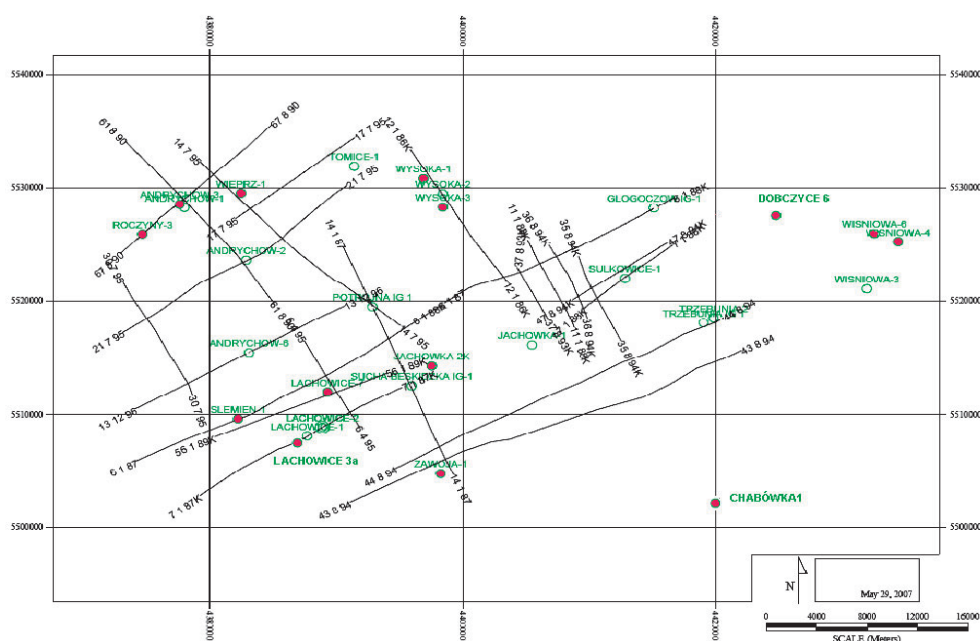
Fig. 1. Schemat położenia otworów, w których wykonano obliczenia parametrów sprężystych na tle zaznaczonych profili sejsmicznych. Wybrane do interpretacji otwory zaznaczono kolorem czerwonym
