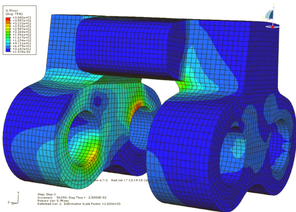
Rys. 7. Warstwie naprężeń Hubera-Misesa w zabieraku obciążonym obwodowo asymetrycznie [MPa]
