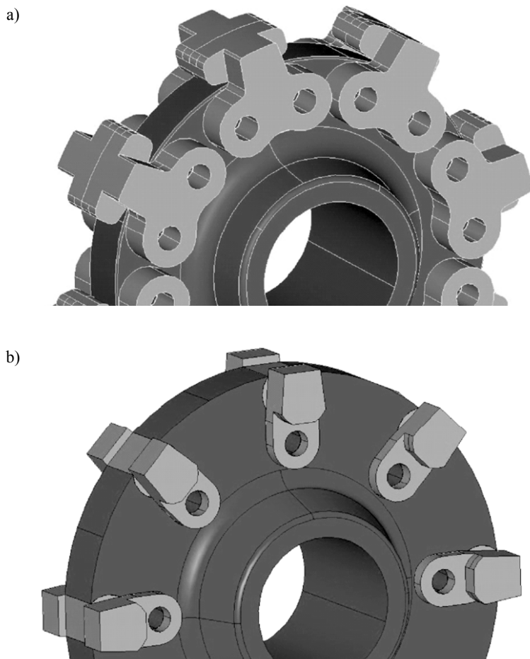
Rys. 3. Połączenie zabieraka z kołem — wersja II i wersja III
