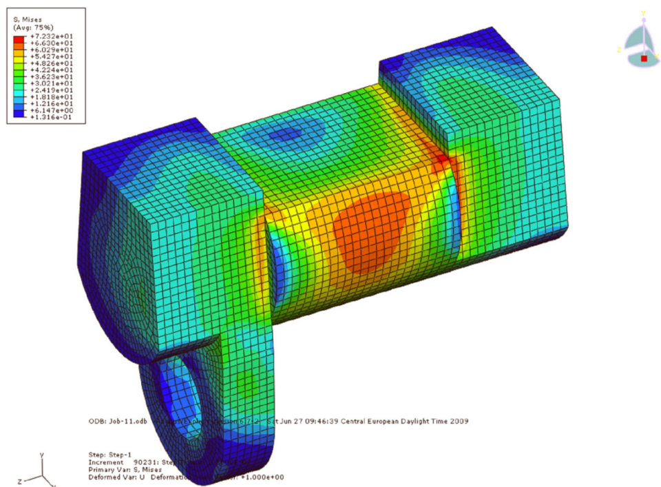
Rys. 8. Warstwyce naprężeń Hubera-Misesa w zabieraku obciążonym obwodowo symetrycznie [MPa]
