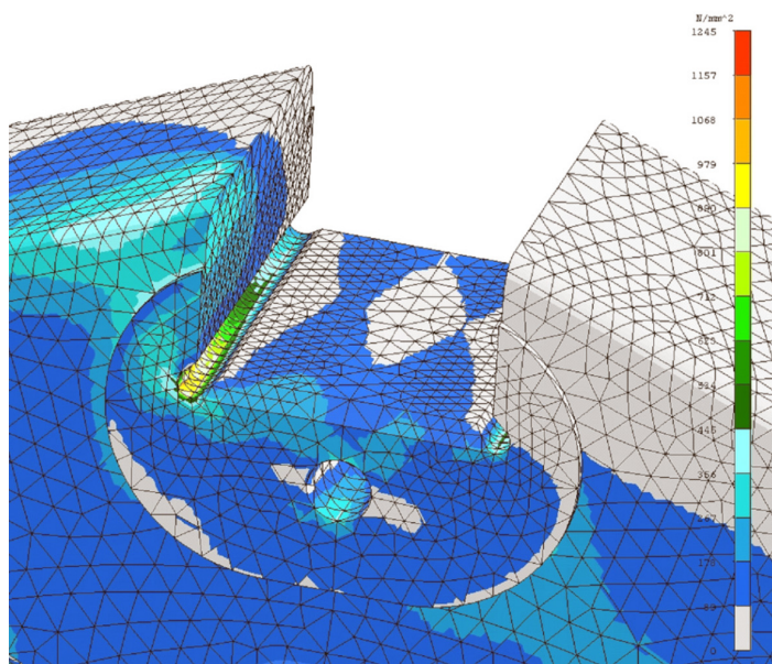
Rys. 6. Warstwiec naprężeń Hubera-Misesa koła zabierakowego obciążonego obwodowo asymetrycznie w [MPa] — koncentracja naprężeń w rowku zabierakowym
