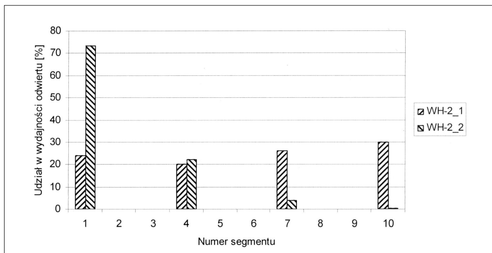
Rys. 12. Zmiany wydatku przepływu w segmentach otworów horyzontalnych WH-2_1 i WH-2_2
