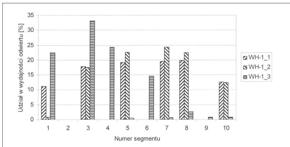
Rys. 11. Zmiany wydatku przepływu w segmentach otworów horyzontalnych WH-1_1 –WH-1_3
