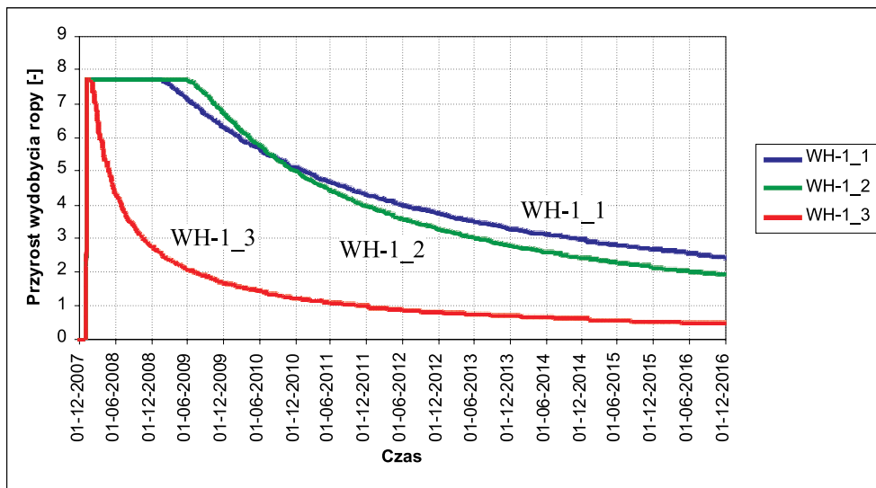
Rys. 9. Względne wydobyte z otworów poziomych WH-1_1 –WH-1_3
