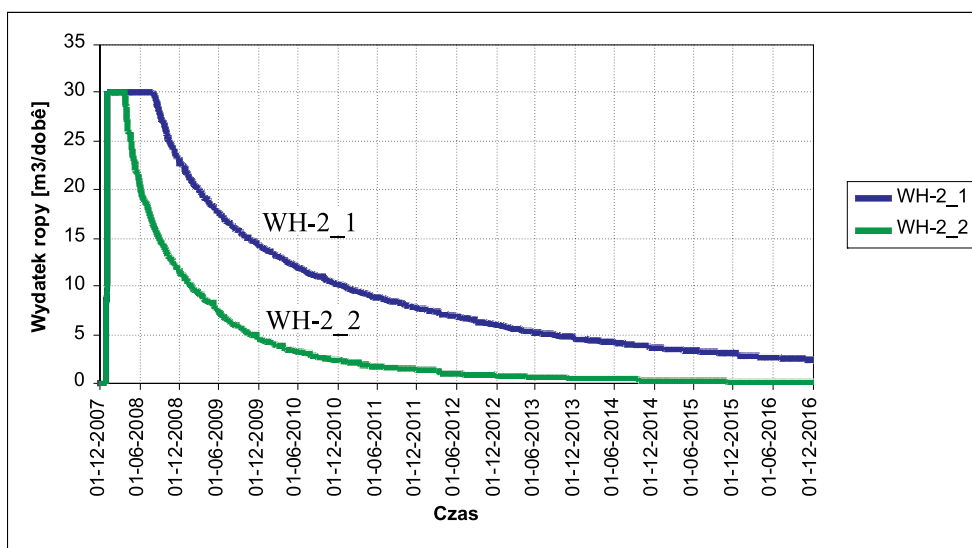
Rys. 4. Zmiany wydajności w czasie w odwiertach WH-2_1 i WH-2_2
