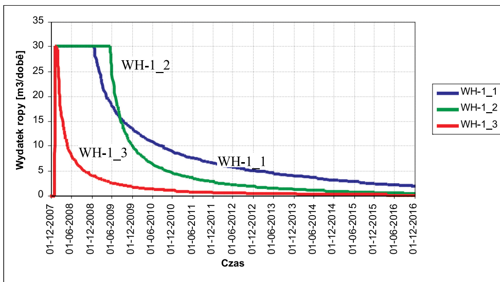
Rys. 3. Zmiany wydajności w czasie w odwiertach WH-1_1 –WH-1_3
