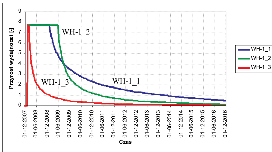
Rys. 5. Względna wydajność otworów horyzontalnych WH-1_1 –WH-1_3
