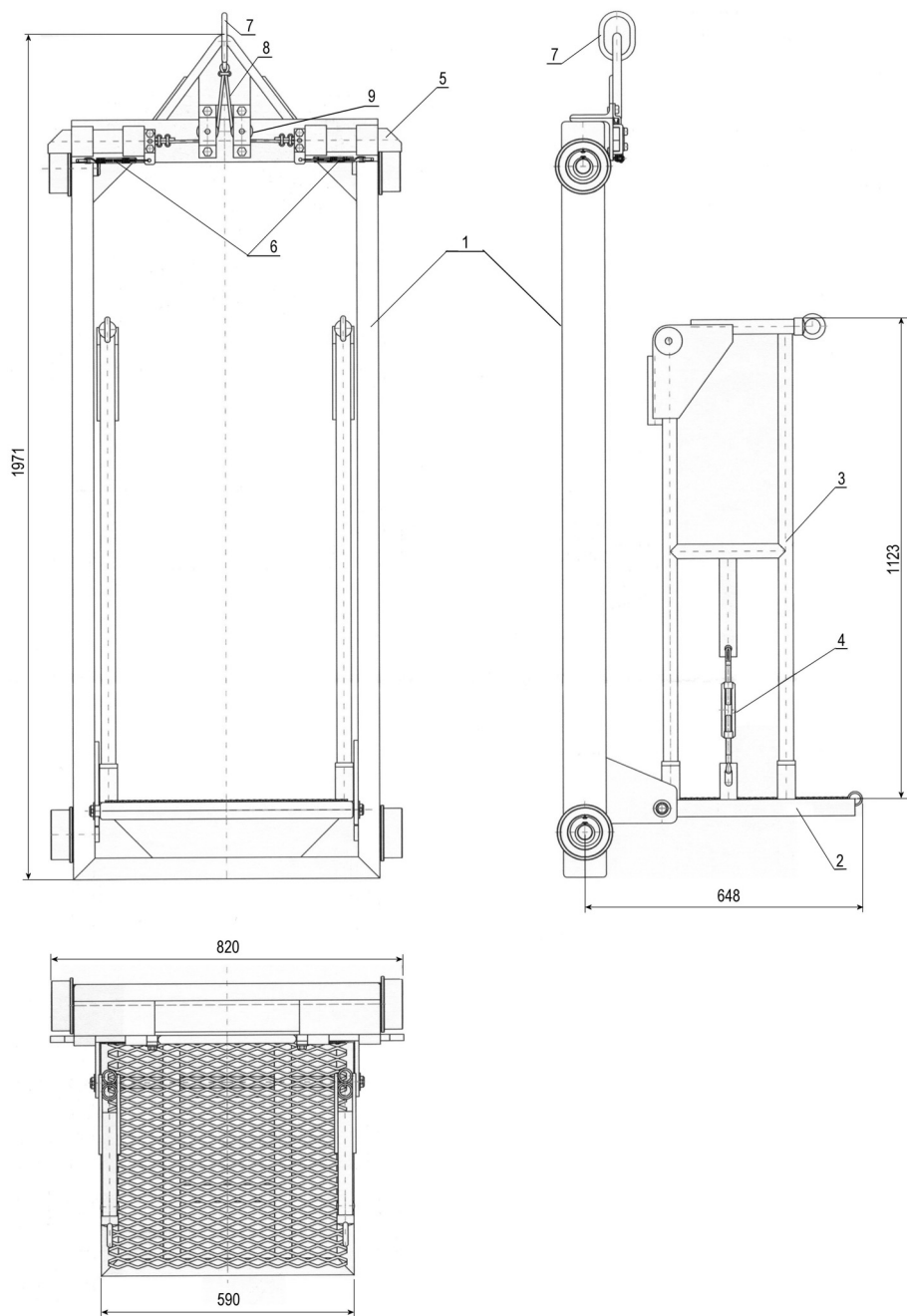
Rys. 2. Pomost roboczy z wózkiem. 1 – wózek, 2 – pomost, 3 – barierka, 4 – śruba rzymska, 5 – rygiel, 6 – sprężyny rygli, 7 – ucho do mocowania liny do wciągarki, 8 – linka spinająca rygle, 9 – kółeczka prowadzące linkę spinającą rygle
