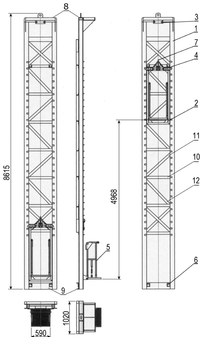
Rys. 1. Mostek do rurowania wraz z ramą nośną. 1 – rama nośna, 2 – wózek jezdny z pomostem, 3 – uchwyty do mocowania wciągarki, 4 – mechanizm ryglujący, 5 – barierka, 6 – ograniczniki, 7 – ucho do mocowania, 8 – dwuteownik, 9 – ceownik, 10, 11 i 12 – kątowniki
