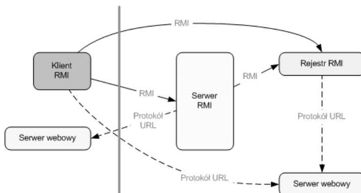
Rys. 3. Działanie rozproszonej aplikacji wykorzystującej rejestr RMI [5]
