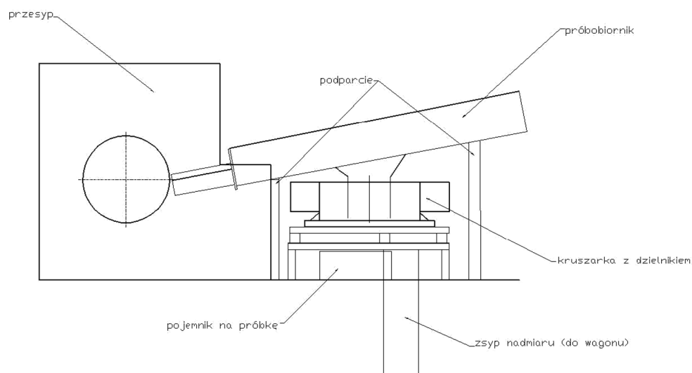
Rys. 9. System poboru próbki z przesypu, z kruszarką dwuwalcową
