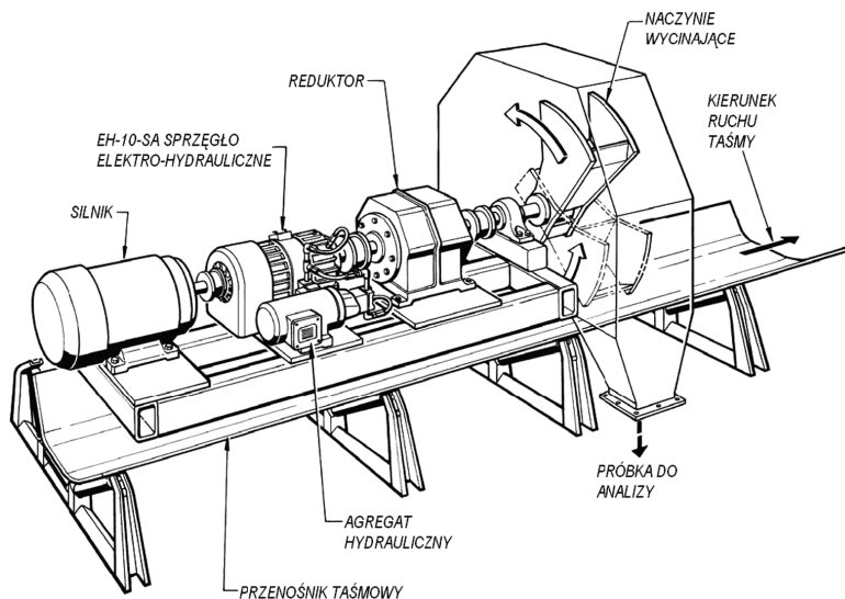
Rys. 3. Próbobiórnik pobierający w poprzek taśmy z ruchem obrotowym naczynia, produkcja Force Control
