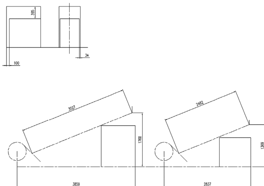
Rys. 14. Porównanie obrysów kruszarek KW-240 KOMAG z najczęściej dotąd stosowaną (ilustracja górna) oraz porównanie gabarytów systemów poboru próbki z przesypu, z zastosowaniem kruszarki KW-240 KOMAG (z prawej) oraz najczęściej dotąd stosowanej (z lewej)
