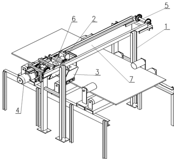
Rys. 10. Próbbiornik PMSN KOMAG, najmniejszy ze znanych obecnie próbbiorników pobierających próbkę z taśmociągu w ruchu, w poprzek taśmy
