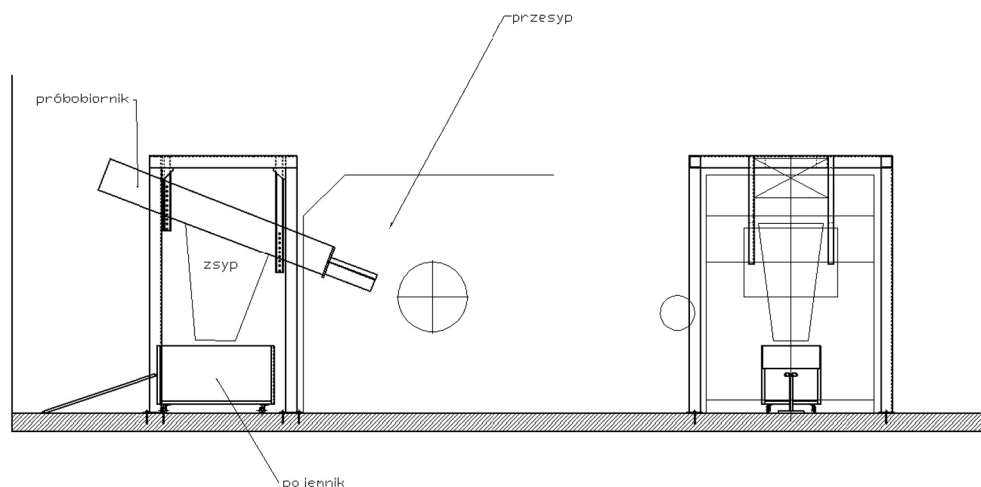
Rys. 8. System poboru próbki z przesypu, bez kruszarki
