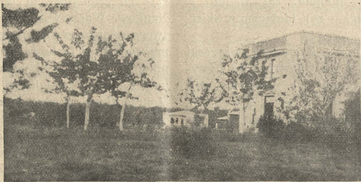
OGÓLNY WIDOK OBSERWATORIUM MAGNETYCZNEGO W ŚWIDRZE; W GŁĘBI DREWNIANY BUDYNEK DO POMIARÓW BEZWZGLĘDNYCH I MUROWANY DLA PRZYRZĄDÓW SAMOPISZĄCYCH.
