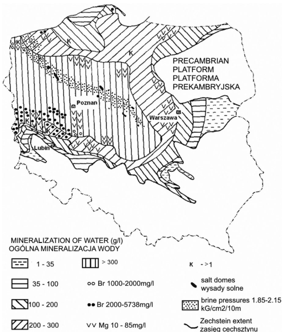
Fig. 7. Hydrochemiczna mapa cechsztynu (za Bojarska &amp; Bojarski 1981)
