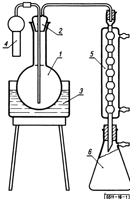
Rys. 1. Zestaw do przygotowania wypełnienia kolumny
