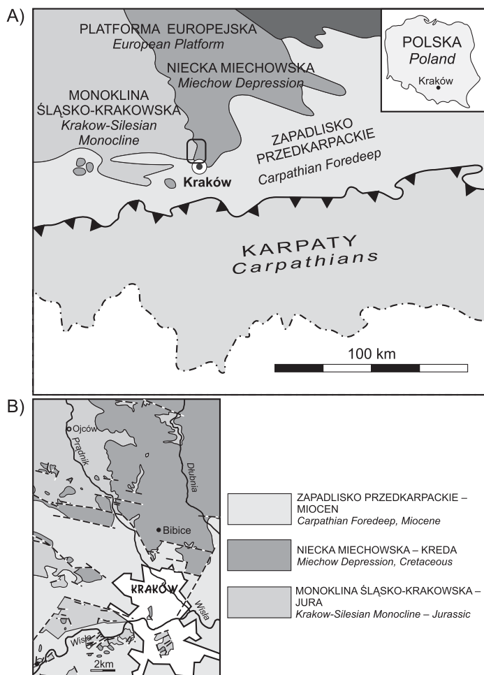
Fig. 1. A) Mapa tektoniczna Platformy Europejskiej, zapadliska przedkarpackiego i Karpat zewnętrznych – lokalizacja obszaru badań, B) mapa geologiczna osadów mezozoicznych regionu krakowskiego (Gradziński 1972)
