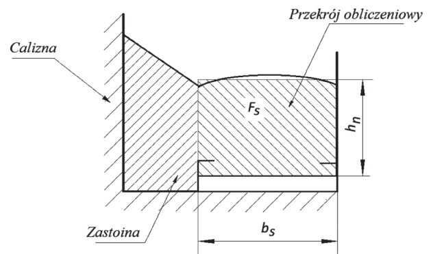
Rys. 4. Rzeczywisty i zastępczy przekrój poprzeczny urobku na rynnach ścianowego przenośnika zgrzeblowego
