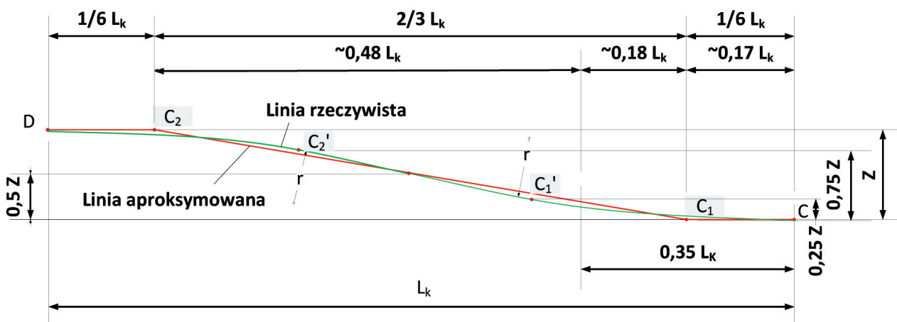
Rys. 6. Zastąpienie rzeczywistej linii krzywizny przenośnika na odcinku zawrębiania kombajnu linią prostą C_1-C_1'-C_2
