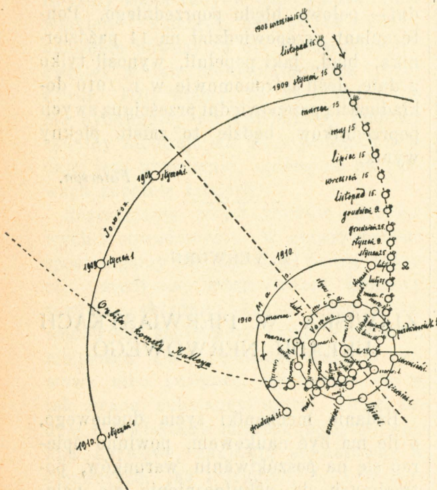
Wyznaczenie drogi komety Halleya dla jej przyszłego powrotu oraz położenie planet w r. 1910.
