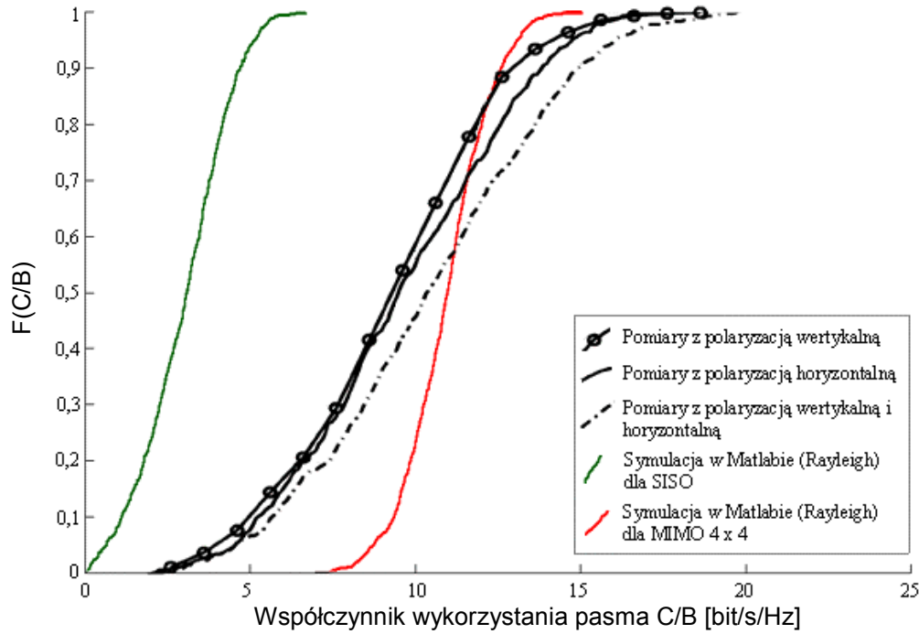
Rys. 5. Dystrybuanta współczynnika wykorzystania pasma w pikokomórce dla układów anten o różnej polaryzacji [12]
