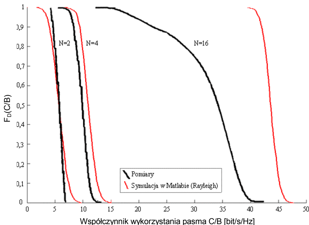
Rys. 9. Funkcja dopełniająca dystrybucyjną współczynnika wykorzystania pasma dla różnych układów antenowych [2]
