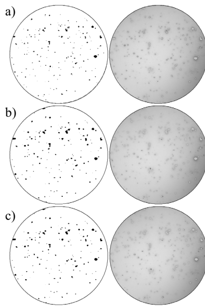
Rys. 11. Obraz test2 , dwuprzebiegowo: a) Bernsen; b) PV ( half ); c) PV ( valley )
