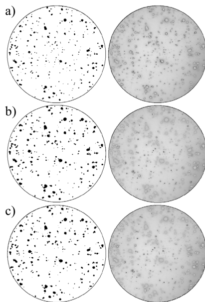
Rys. 13. Obraz test3 , maska 75 \times 75 : a) Bernsen; b) PV ( half ); c) PV ( valley )
