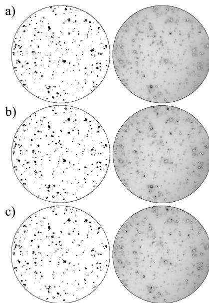
Rys. 12. Obraz test3 , maska 15 \times 15 : a) Bernsen; b) PV ( half ); c) PV ( valley )
