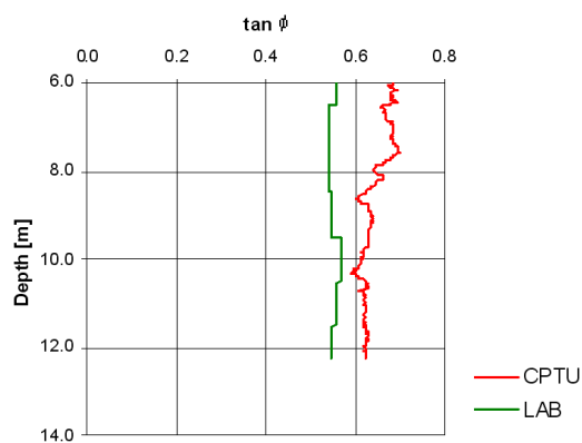
Rys. 13. Porównanie interpretacji wyników badań laboratoryjnych i CPTU Glava-clay Stjoldal
