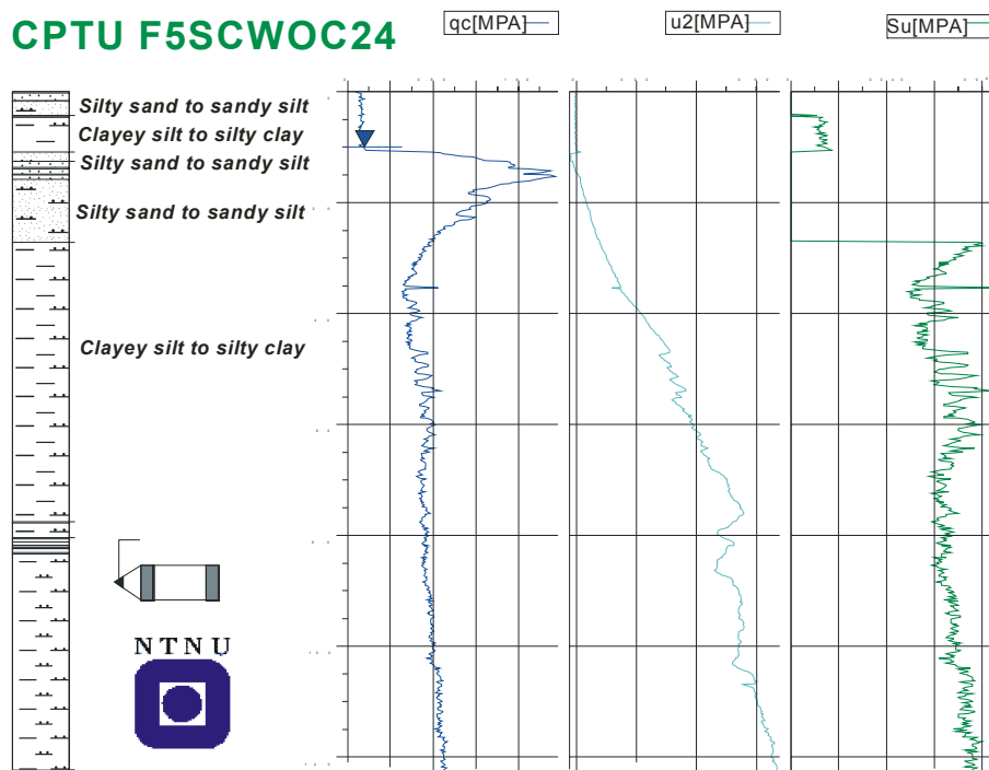
Rys. 12. Wynik sondowań CPTU Glava-clay Stjoldal
