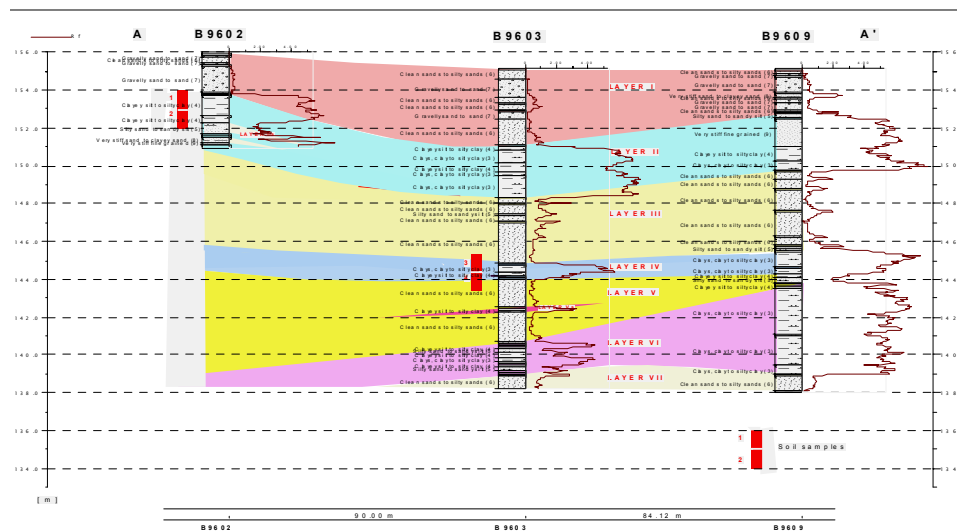
Rys. 19. Interpretacja wyników sondowań CPTU wykres oporu na pobocznicę R_f [MPa]
