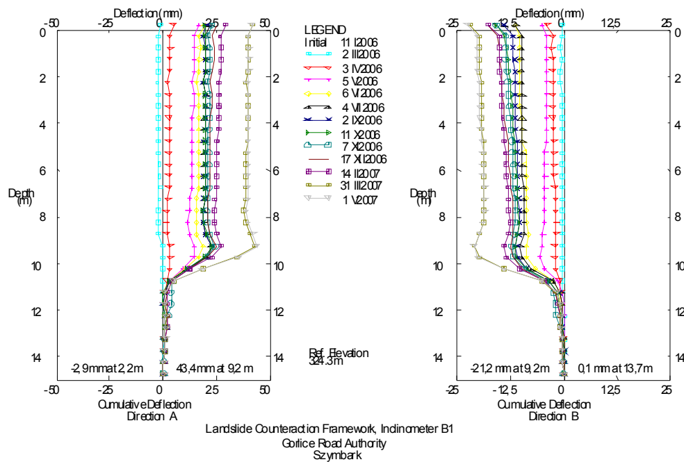
Rys. 3. Pomiary przemieszczeń wgłębnych
