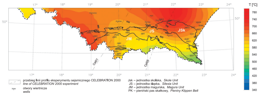
Fig. 4. Rozkład temperatur na granicy Moho na obszarze Karpat polskich
