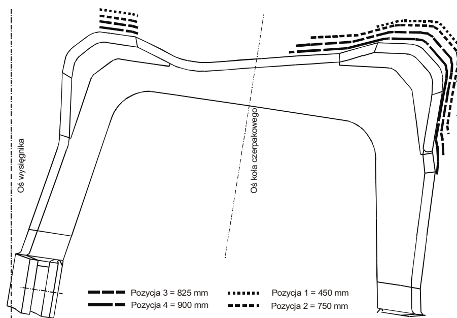
Rys. 7. Czerpak asymetryczny, ruch wysięgnika w prawą stronę
