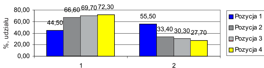
Rys. 8. Procentowy udział krawędzi tnących naroża prawego naroża 1 i lewego 2 czepaka symetrycznego przy ruchu wysięgnika w prawą stronę; 1 – naroże prawe, 2 – naroże lewe
