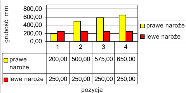
Rys. 10. Grubość zabieranego wióra dla prawego i lewego naroża czepaka symetrycznego
