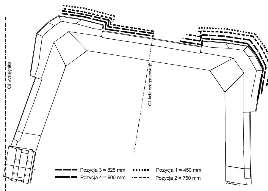
Rys. 6. Czerpak symetryczny, ruch wysięgnika w prawą stronę
