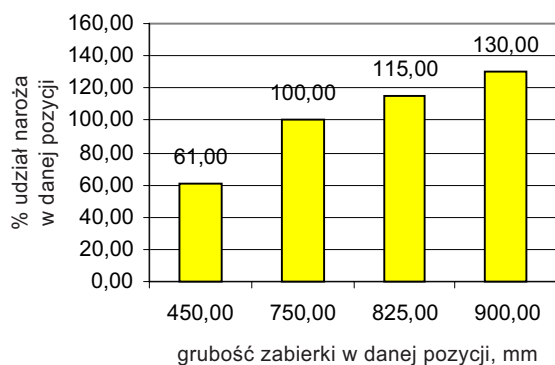
Rys. 12. Udział krawędzi tnących w odniesieniu do naroża lewego dla czepaka asymetrycznego
