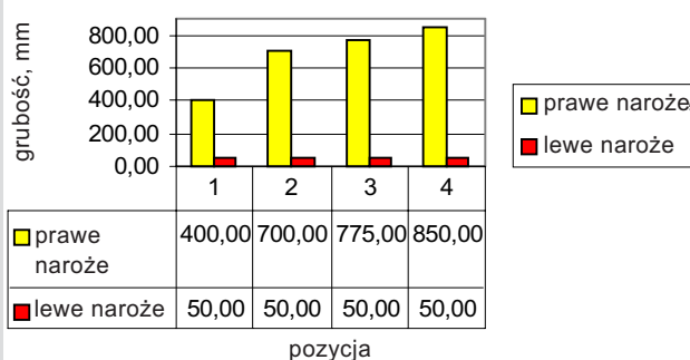
Rys. 11. Grubość zabieranego wióra dla prawego i lewego naroża czepaka symetrycznego
