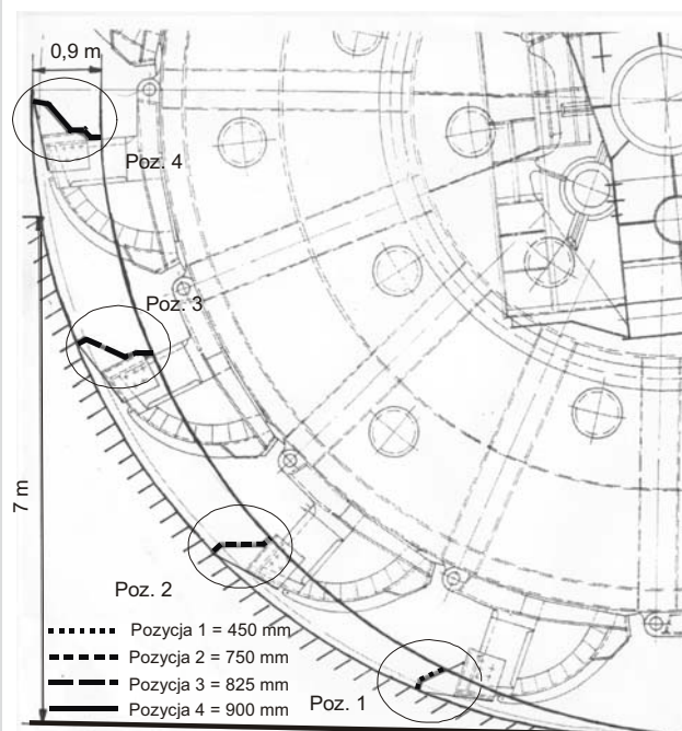
Rys. 3. Poszczególne fazy wchodzenia czerpaka w caliznę
