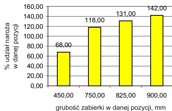
Rys. 13. Udział krawędzi tnących w odniesieniu do naroża lewego dla czepaka symetrycznego
