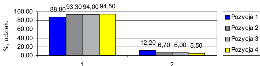
Rys. 9. Procentowy udział krawędzi tnących naroża prawego naroża 1 i lewego 2 czepaka asymetrycznego przy ruchu wysięgnika w prawą stronę; 1 – naroże prawe, 2 – naroże lewe
