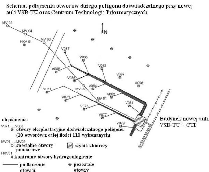
Rys. 3. Plan sytuacyjny z rozmieszczeniem poszczególnych otworów na dużym poligonie badawczym
