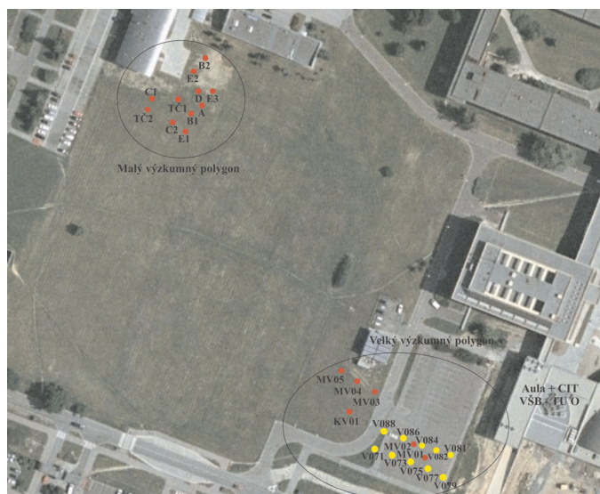
Rys. 4. Widok na planie poziomym usytuowania otworów badawczych małego i dużego poligonu badawczego względem zabudowań VSB-TU Ostrawa
