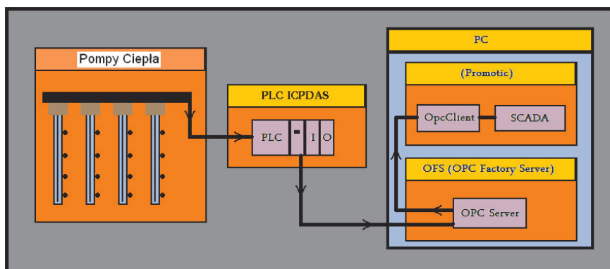
Rys. 7. Schemat ideowy systemu pomiarowego
