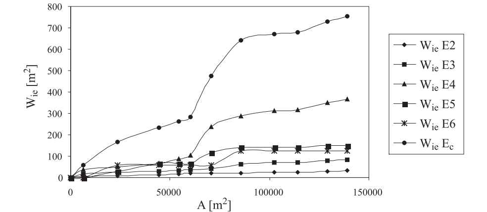
Rys. 2. Wykres zmiany wskaźnika intensywności energii w funkcji zwiększającego się pola powierzchni dokonanej eksploatacji dla ściany 62
