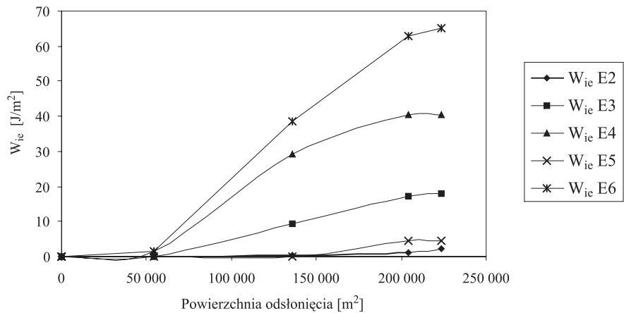
Rys. 10. Wykres zmiany wskaźnika intensywności energii w funkcji zwiększającego się pola powierzchni dokonanej eksploatacji dla ściany 44
