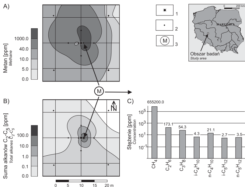
Fig. 2. Rozkład stężeń metanu (A), sumy alkanów C 2 -C 5 (B), skład cząsteczkowy alkanów w punkcie M (C) – rejon odwiertu W-29 (PMG Wierchowice): 1 – badany odwiert, 2 – punkt pomiarów geochemicznych, 3 – miejsce maksymalnego stężenia alkanów
