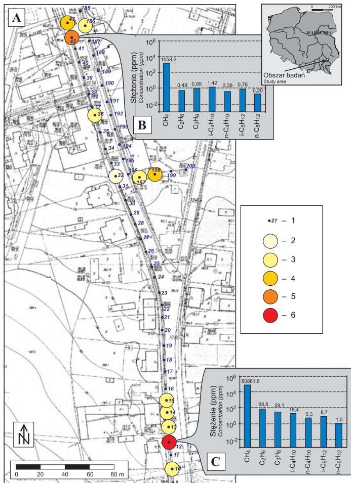
Fig. 4. Prawdopodobne strefy nieuszczelności gazociągu niskiego ciśnienia położonego wzdłuż ul. Mickiewicza w Leżajsku (A), skład cząsteczkowy alkanów w miejscu o wysokim (B) i bardzo wysokim (C) prawdopodobieństwie występowania nieuszczelności: 1 – punkt pomiarów geochemicznych, 2–6 – prawdopodobieństwo występowania nieuszczelności: 2 – potencjalne, 3 – niskie, 4 – średnie, 5 – wysokie, 6 – bardzo wysokie
