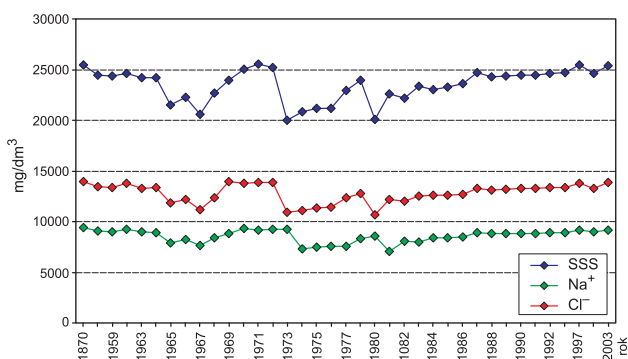
Fig. 2. Mineralizacja (SSS) oraz zawartości \text{Na}^+ i \text{Cl}^- w wodach chlorkowych z ujęcia Krakus
