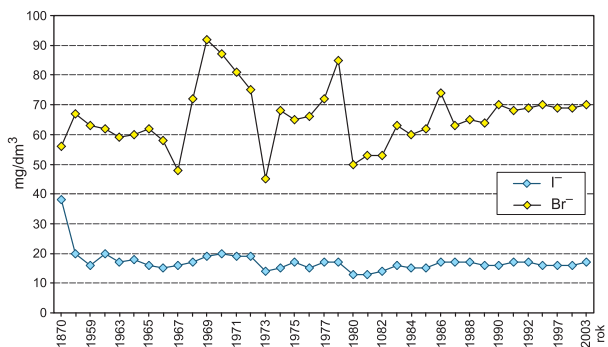
Fig. 3. Zawartość \text{I}^- i \text{Br}^- w wodach chlorkowych z ujęcia Krakus
