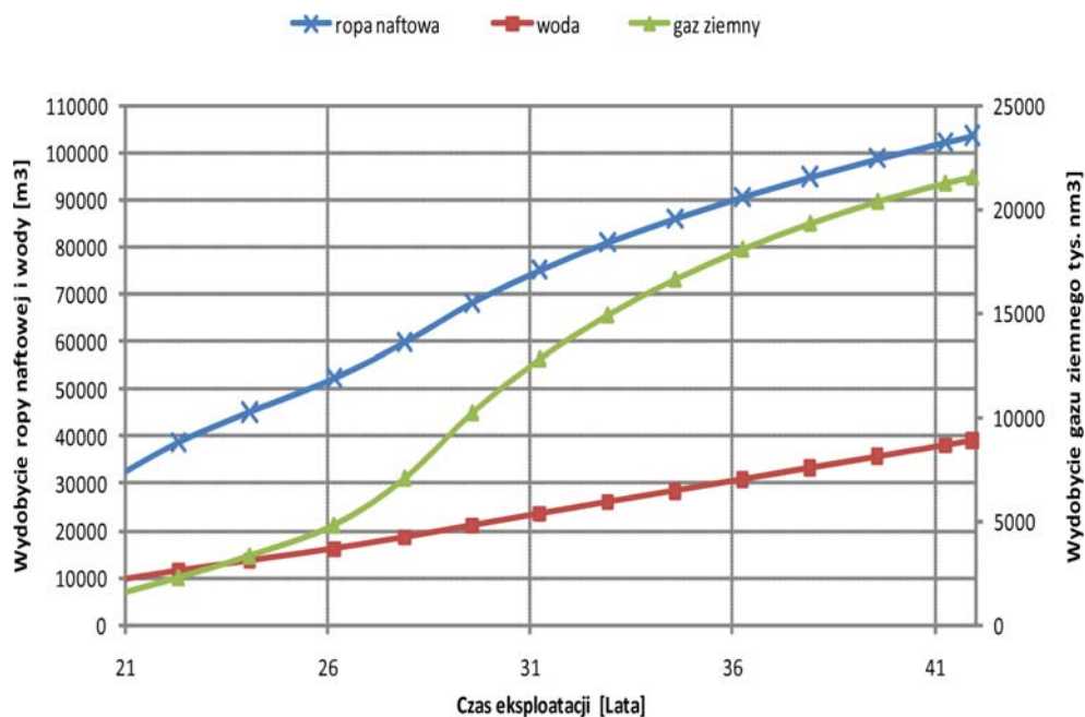
Rys. 3. Skumulowane wydobywanie płynów złożowych – wariant II
