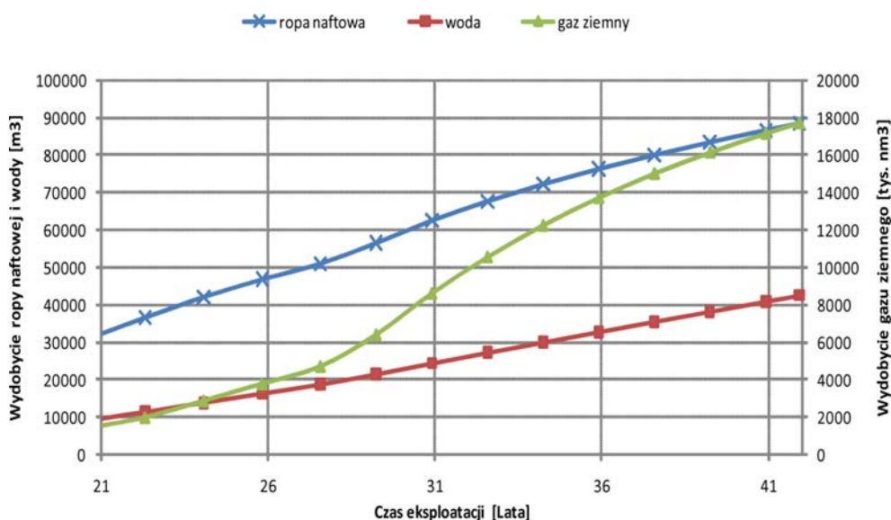
Rys. 2. Skumulowane wydobywanie płynów złożowych – wariant I
