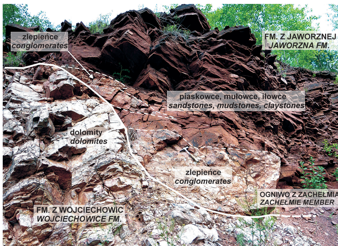
Fig. 20. Zachodnia krawędź kopalnej dolinki/wąwozu, wyłobionej w dolomitach formacji z Wojciechowic. Jej wypełnienie stanowią utwory formacji z Jaworznej, wykształcone jako zlepieńcowate osady sływów gruzowo-błotnych, zachowane w postaci tarasów (ogniwo z Zachelmia) oraz piaskowcowo-mułowcowo-iłowcowe osady okresowych strumieni i jezior typu playa. Wschodnia ściana kamieniołomu Zachelmie (Fig. 1B, pkt 12), fot. Z. Złonkiewicz • Western wall margin of a palaeo valley/ravine, cut in dolomites of the Wojciechowice Formation. It's filled with the Jaworzna Formation represented by conglomerate deposits of mud-debris flows forming terraces (Zachelmie Member), as well as sandstone-mudstone-clay deposits of temporary creeks and playa-like ponds. Eastern wall of Zachelmie quarry (Fig. 1 B, stop 12), photo Z. Złonkiewicz
