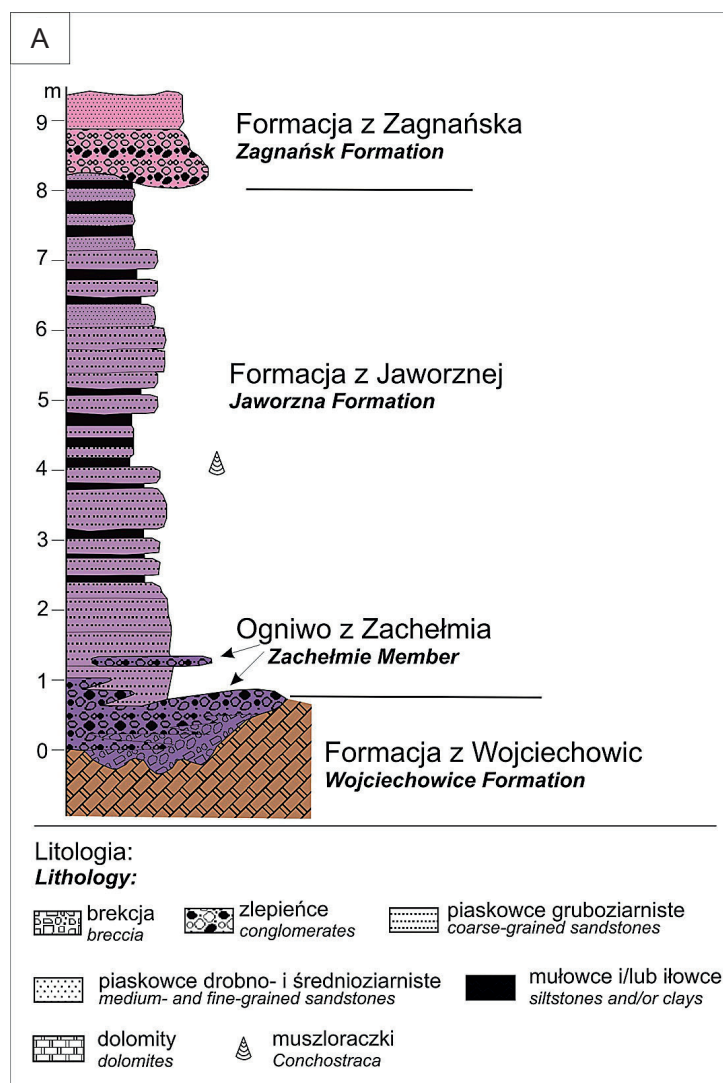
Fig. 4. Profil osadów dolnego triasu (Fig. 1B, pkt 13), leżących niezgodnie na dolomitach dewonu we wschodniej ścianie kamieniołomu Zachełmie, fot. Z. Złonkiewicz. A – według Kuleta et al. (2006), B – według Złonkiewicz & Becker (2015) • Section of the Lower Triassic deposits (Fig. 1B, stop 13), overlying an unconformity surface of the Devonian dolomites in the eastern wall of the Zachełmie quarry, photo Z. Złonkiewicz. A – according to Kuleta et al. (2006), B – according to Złonkiewicz & Becker (2015)
