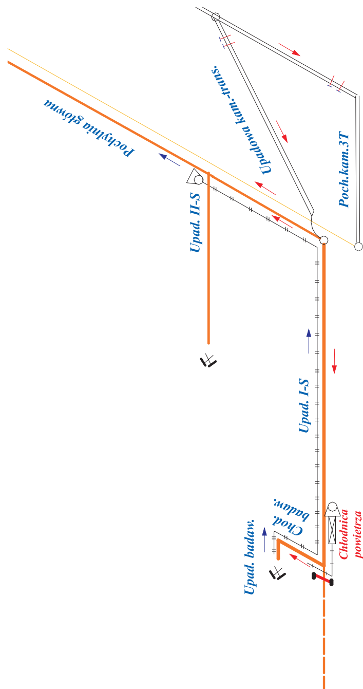
Rys. 1. Schemat ideowy regionu upadowej I-S, chodnika badawczego i upadowej badawczej w pokładzie 407/4 na poziomie 720
