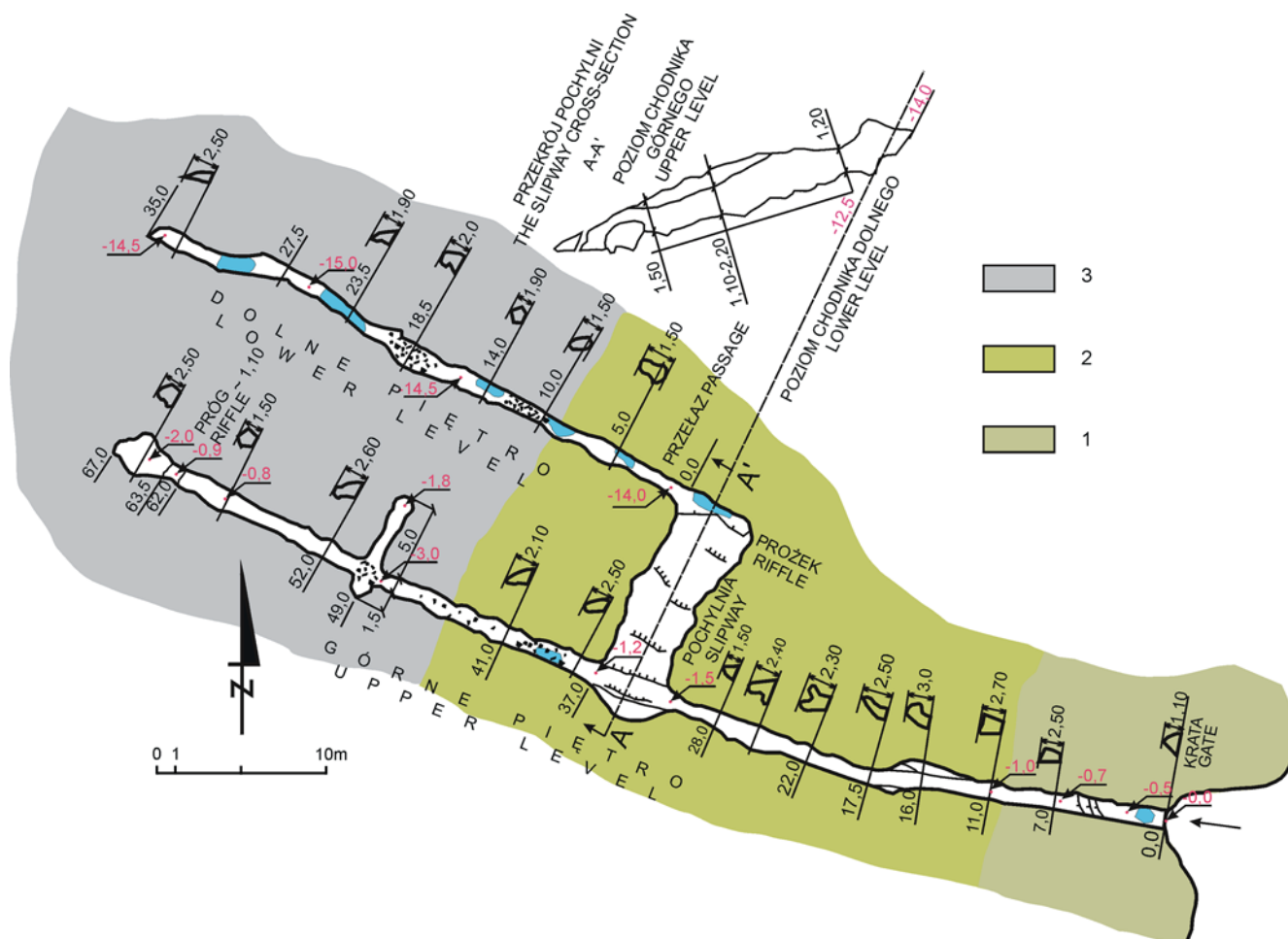
Fig. 12. Plan sztolni w Jarmucie. 1 – zlepienie formacji jarmuckiej (zmienione kontaktowo), 2 – piaskowce formacji jarmuckiej (zmienione kontaktowo), 3 – andezyty (Wojciechowski 1955; Janik 2006, zmieniiony) • Plan of the Jarmuta adit. 1 – conglomerates of the Jarmuta Fm. (contact metamorphosed), 2 – sandstones of the Jarmuta Fm. (contact metamorphosed), 3 – andesites (Wojciechowski 1955; Janik 2006, modified)
