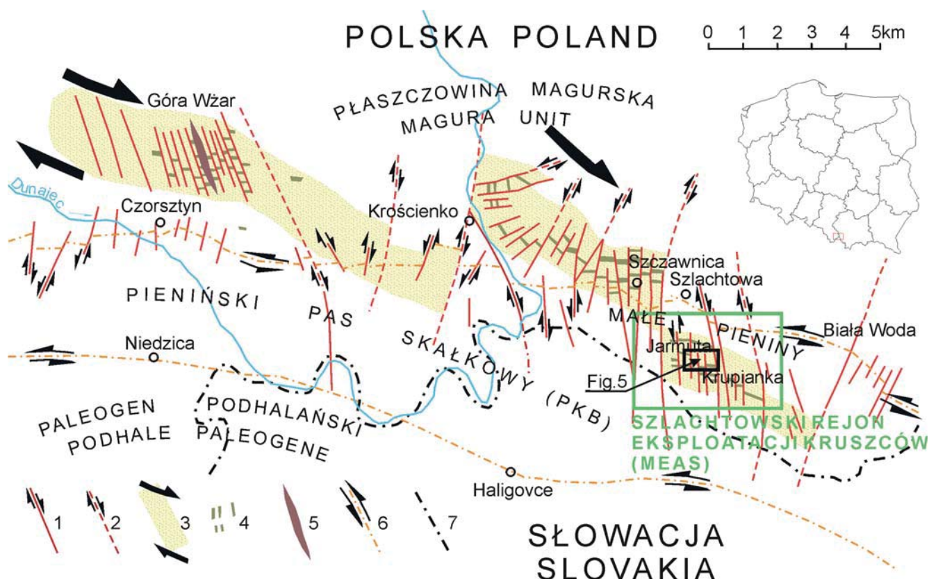
Fig. 6. Szlachtowski rejon eksploatacji kruszców na tle pieninińskiej linii andezytowej (PAL). 1 – poprzeczne uskoki przesuwne prześledzone na powierzchni, 2 – prawdopodobne poprzeczne uskoki przesuwne w podłożu płaszczowiny magurskiej, 3 – PAL z podanym kierunkiem przemieszczenia przesuwczego, 4 – dajki andezytowe starszej generacji, 5 – dajki andezytowe młodszej generacji, 6 – podłużne uskoki przesuwne brzeżne pieninińskiego pasa skałkowego, 7 – granica państw (Birkenmajer, 1996, zmodyfikowany) • Mineral extraction area of Szlachtowa in relation to the Pieniny Andesite Line (PAL), 1 – transversal strike-slip faults traceable at the surface, 2 – supposed transversal strike-slip faults in substratum of the Magura Nappe, 3 – PAL with sense of strike-slip translation marked, 4 – older generation andesite dykes, 5 – younger generation andesite dykes, 6 – longitudinal strike-slip boundary faults, 7 – border of the countries, MEAS – mineral extraction area of Szlachtowa, PKB – Pieniny Klippen Belt (Birkenmajer, 1996, modified)
