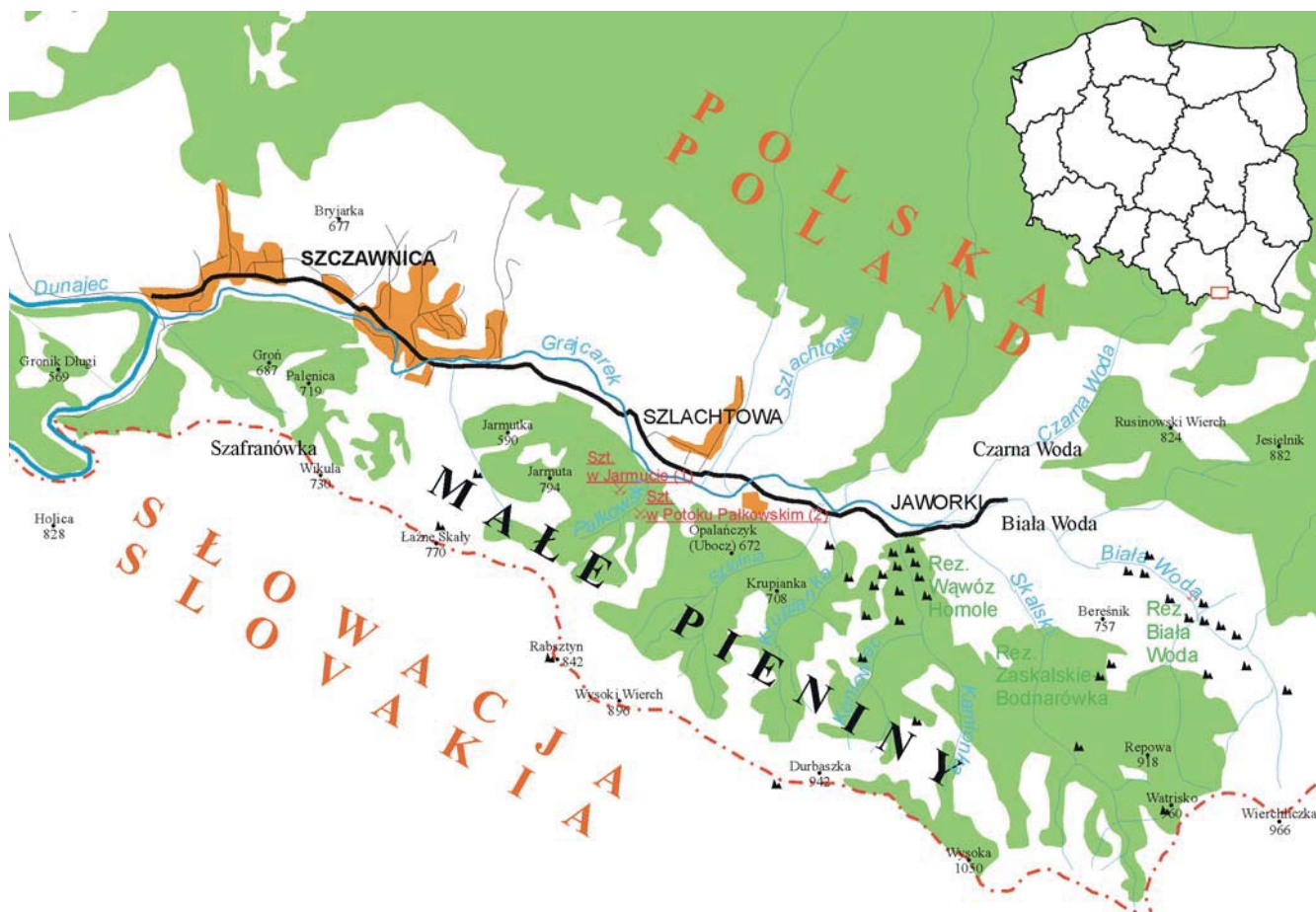
Fig. 2. Topografia Małych Pienin (OPGK w Krakowie, 1993, zmodyfikowany) • Topography of the Małe Pieniny Mts., 1 – Jarmuta adit, 2 – Palkowski stream adit (OPGK in Kraków, 1993, modified)
