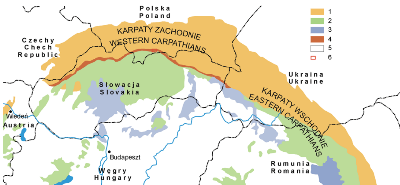
Fig. 3. Szkic tektoniczny regionu karpackiego. 1 – Karpacie zewnętrzne, 2 – Karpacie wewnętrzne, 3 – neogeńskie wulkanity, 4 – pieniński pas skałkowy, 5 – baseny neogeńskie, 6 – pozycja Fig. 5 (Kováč i in., 1998, zmodyfikowany) • Tectonic sketch map of the Carpathian region, 1 – Outer Carpathians, 2 – Inner Carpathians, 3 – Neogene volcanic areas, 4 – Pieniny Klippen Belt, 5 – Neogene basins, 6 – Fig. 5 position (Kováč et al. 1998, modified)
