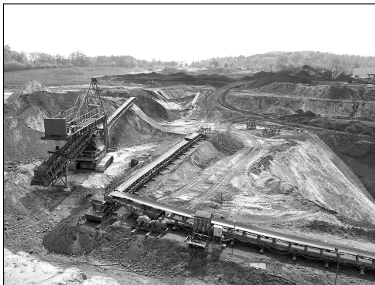
Rys. 3. Eksploatacja odkrywkowa siódła IX stan na rok 2006 [G. Galiniak]
