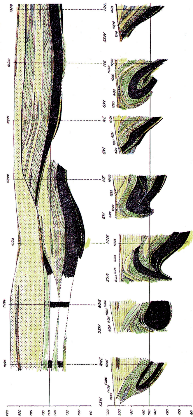
Rys. 1. Przekrój przez złożę węgla brunatnego „Sieniawa” [6]
