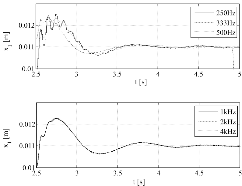
Rys. 17. Położenie obiektu lewitującego dla t \in [t_2, t_3)
