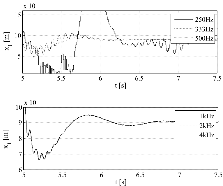
Rys. 18. Położenie obiektu lewitującego dla t \in [t_3, t_4)
