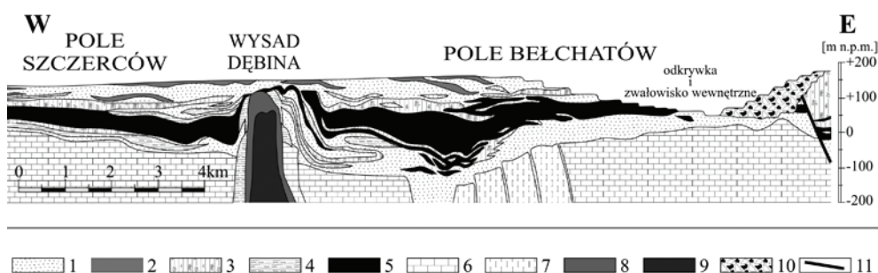
Rys. 2. Przekrój geologiczny przez złoża Belchatów (na podst. [6]): 1 — piaski; 2 — gliny zwałowe; 3 — iły; 4 — mułki; 5 — węgiel brunatny; 6 — wapień; 7 — margle; 8 — czapa gipsowo-anhydrytowa wysadu solnego; 9 — sól kamienna; 10 — zwałowisko wewnętrzne; 11 — główne uskoki tektoniczne
