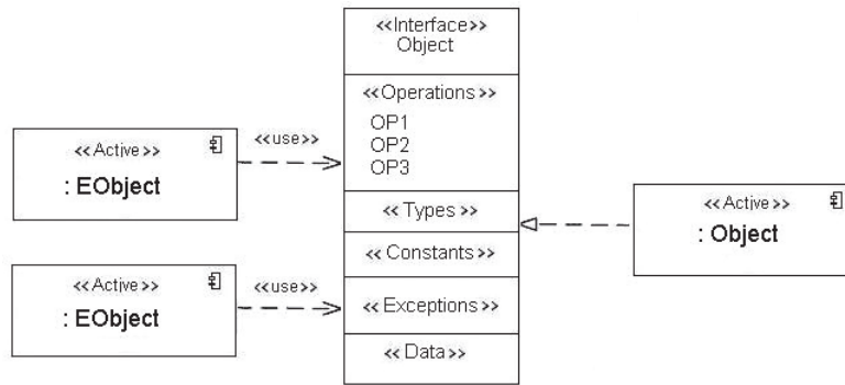
Rys. 6. Konfiguracja przykładowego systemu w HOOD
